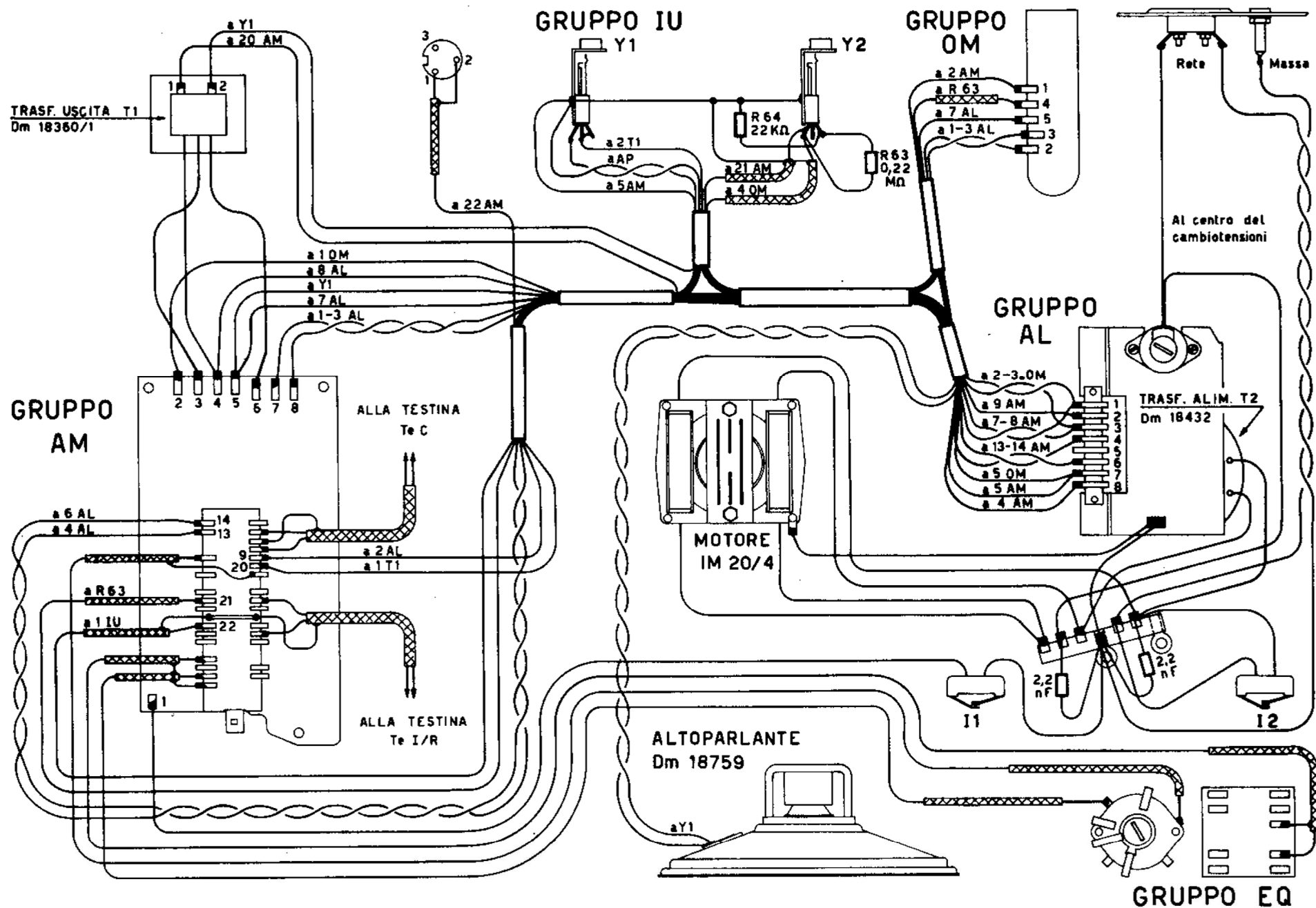
Fig. 4 - Cablaggio
